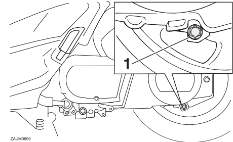
1. Aftapplug versnellingsbakolie
