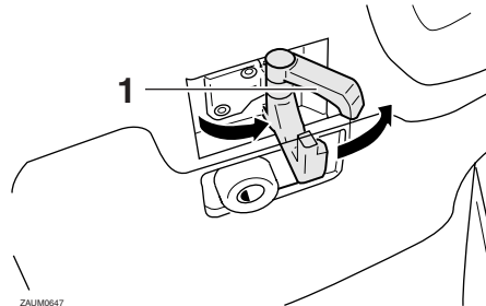
1. Bagagehaak
